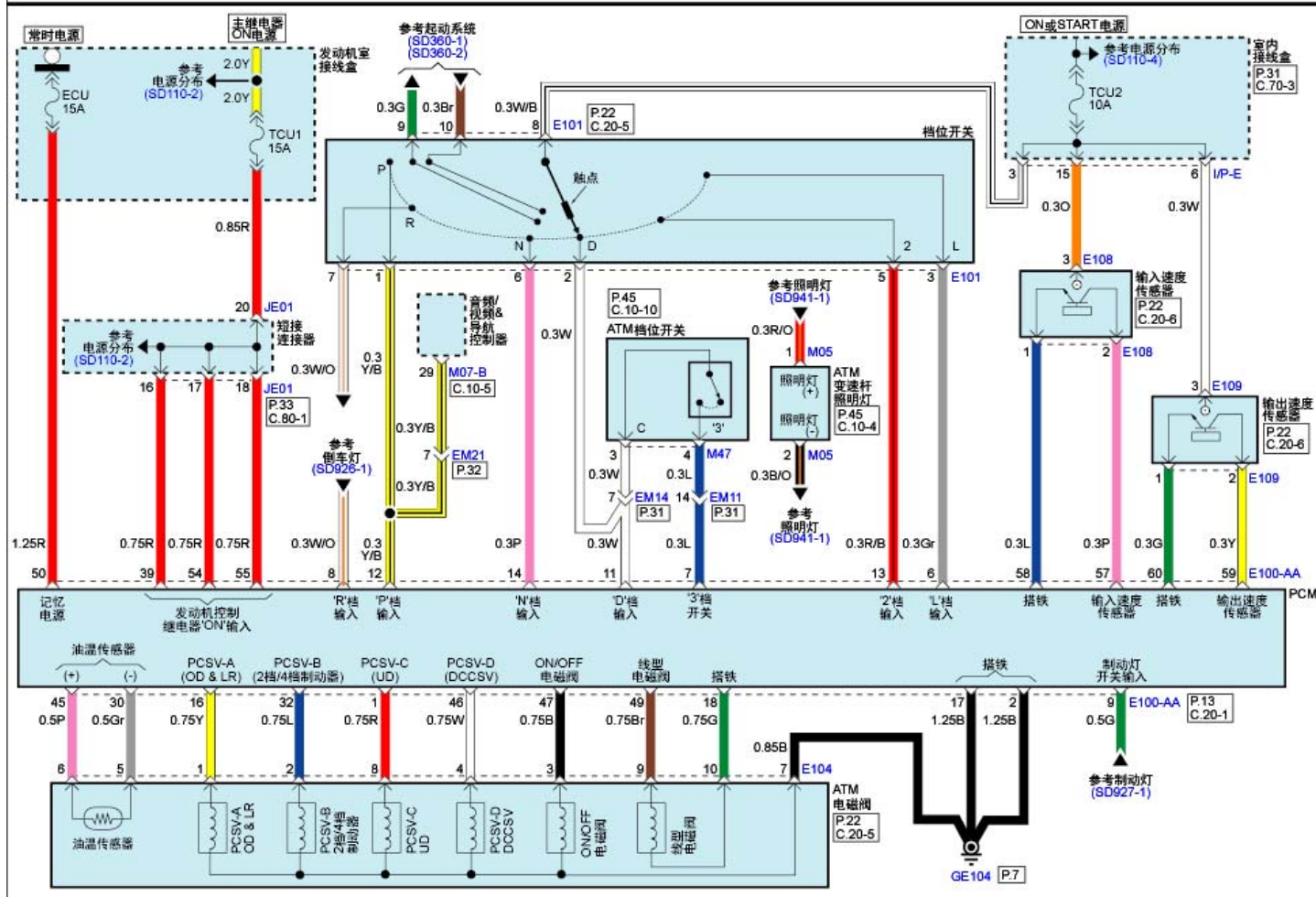
自动变速器控制系统(G4LC : KAPPA 1.4L MPI)(1)
